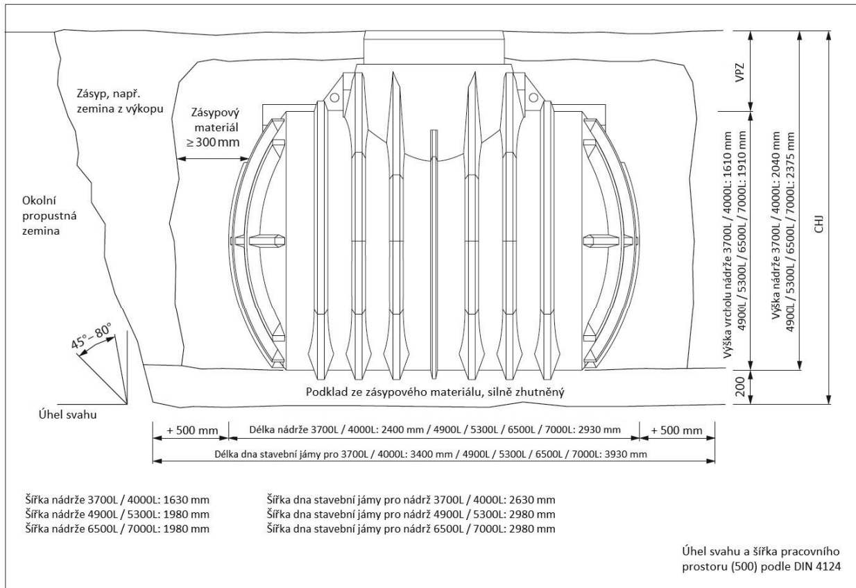
Obr. 2: Montážní velikosti
